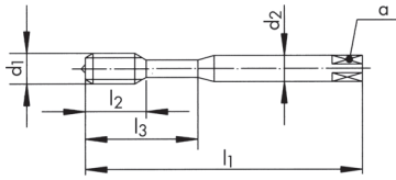
RTS320VS-4 (~DIN371)
