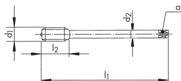
Q460VS-3 (DIN376)
