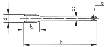
RTS420VS-4 (~DIN376)
