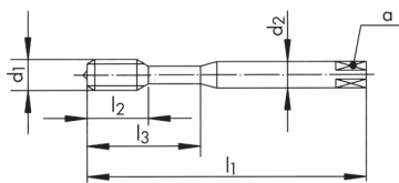
RTS362VS-3 (~DIN371)
